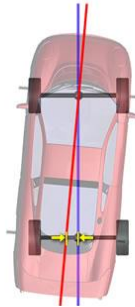
후륜 마이너스 차체 중심선 오프셋
