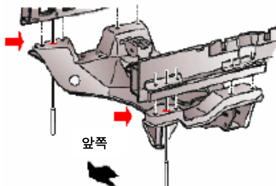
앞쪽 크래들
