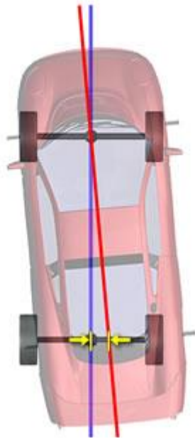
후륜 플러스 차체 중심선 오프셋
